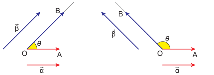
Σχήμα Γωνία δύο διανυσμάτων
