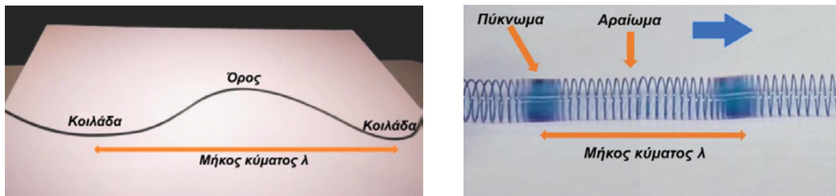
Εικόνα 6.1.5: Εγκάρσιο κύμα σε σχοινί και διάμηκες κύμα σε ελατήριο κυματισμών
