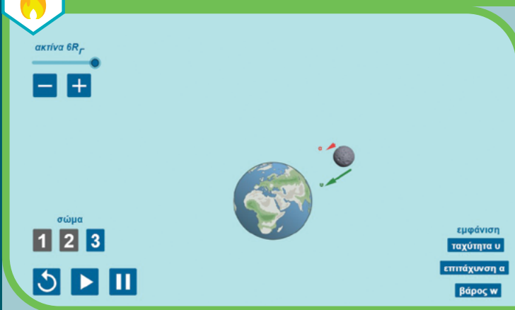
Εικόνα 4.3.1: Αστεροειδής που πλησιάζει τη Γη
