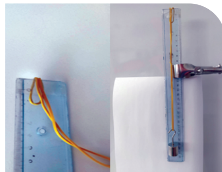
Εικόνα 2.1.3: Πειραματική διάταξη
