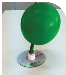
Εικόνα 2.2.7: Ιδιοκατασκευή hovercraft
