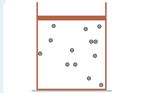
Εικόνα 2.3.10: Κίνηση των μορίων του αερίου
