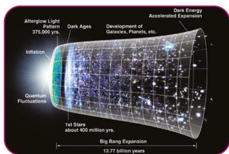
Χρονοδιάγραμμα ζωής του Σύμπαντος μετά τη «Μεγάλη Έκρηξη».
