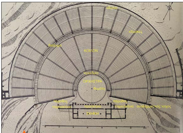
Εικόνα 4. Σχεδιαστική κάτοψη του θεάτρου της Επιδαύρου. Φαίνονται τα βασικά μέρη του αρχαίου ελληνικού θεάτρου: κείμεναι, ορχήστρα, σκηνή, παρασκήνια, πάροδος.
