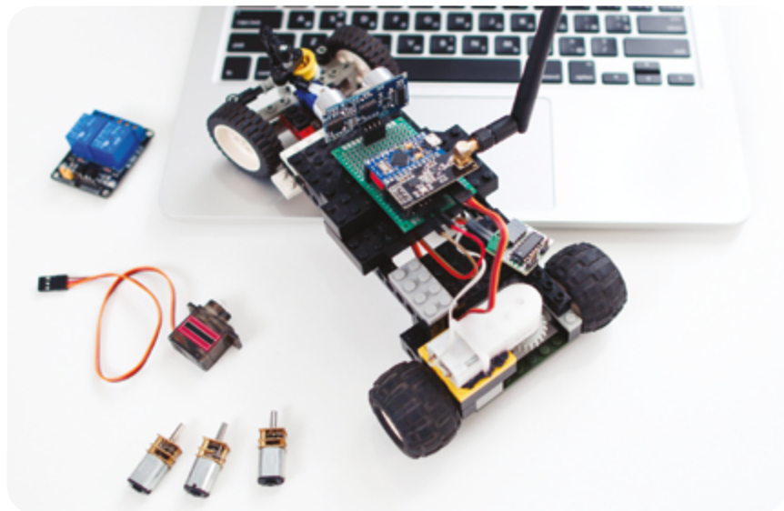
Εικόνα 2. Ρομπωτικό όχημα ελεγχόμενο από μικροελεγκτή τύπου micro:bit
